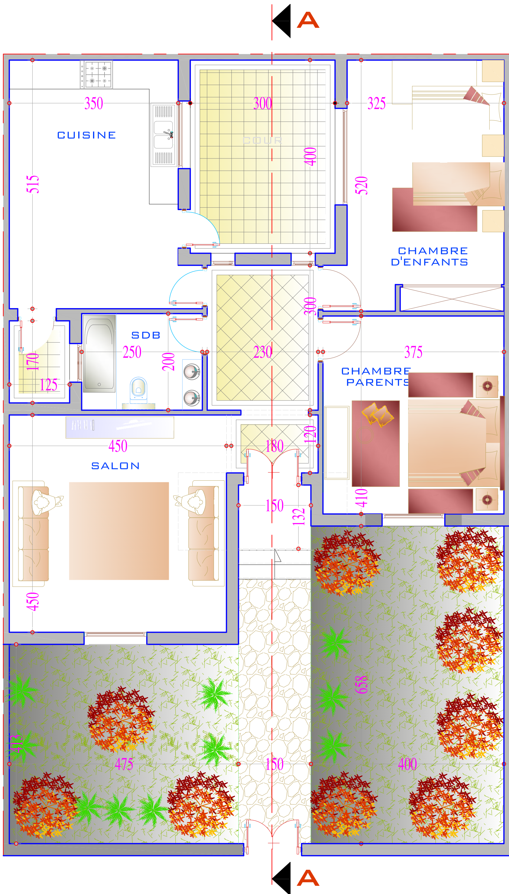
PLAN RDC ECHELLE 1/100
