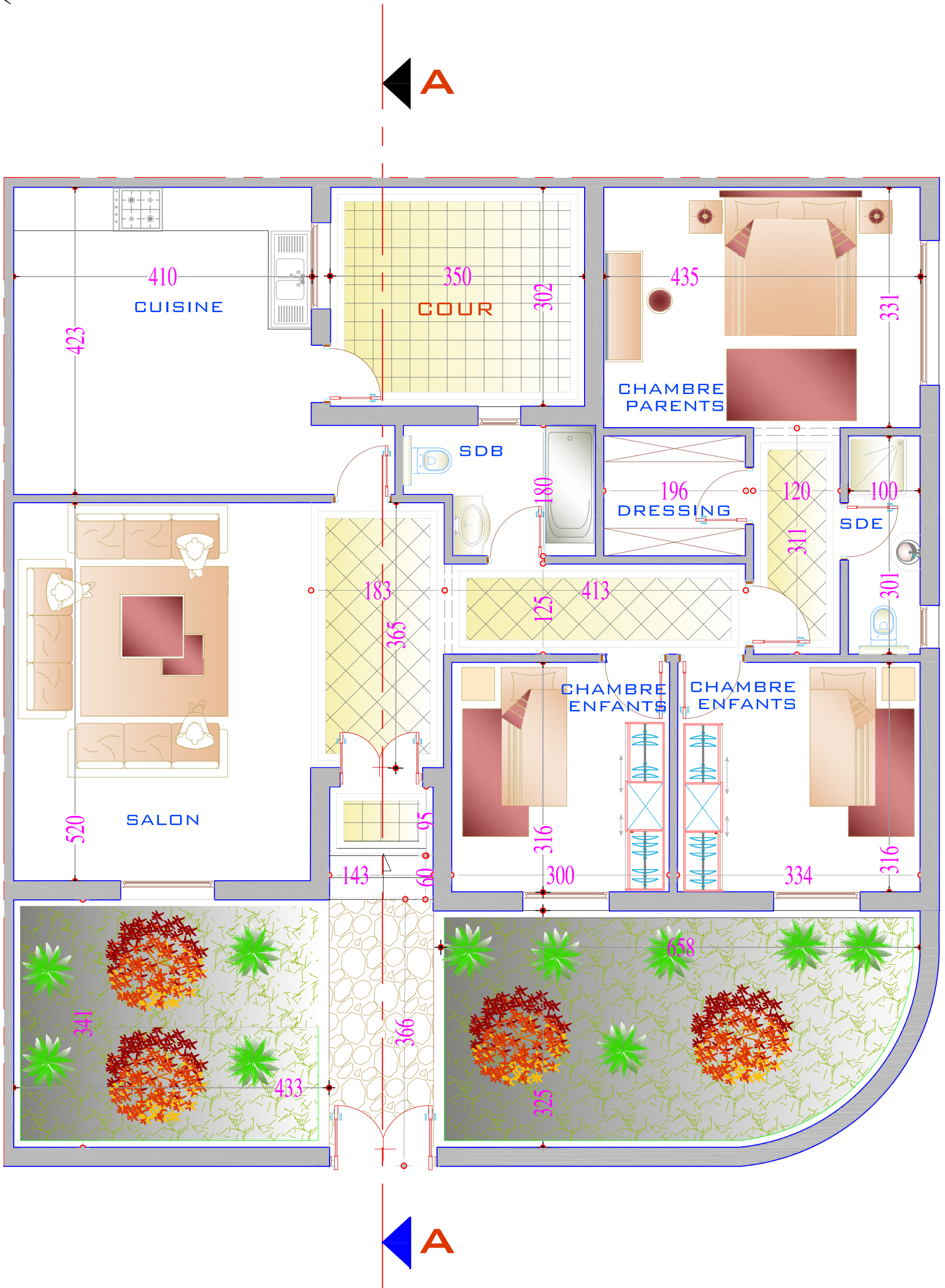
PLAN RDC ECHELLE 1/100
