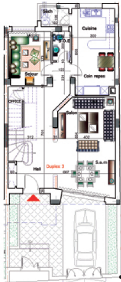
PLAN REZ DE CHAUSSEE
