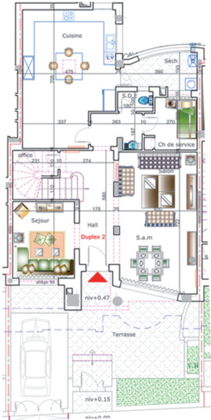
PLAN REZ DE CHAUSSEE
