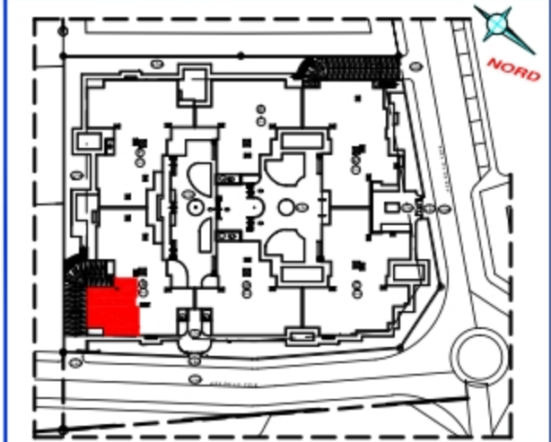
PLAN MASSE
